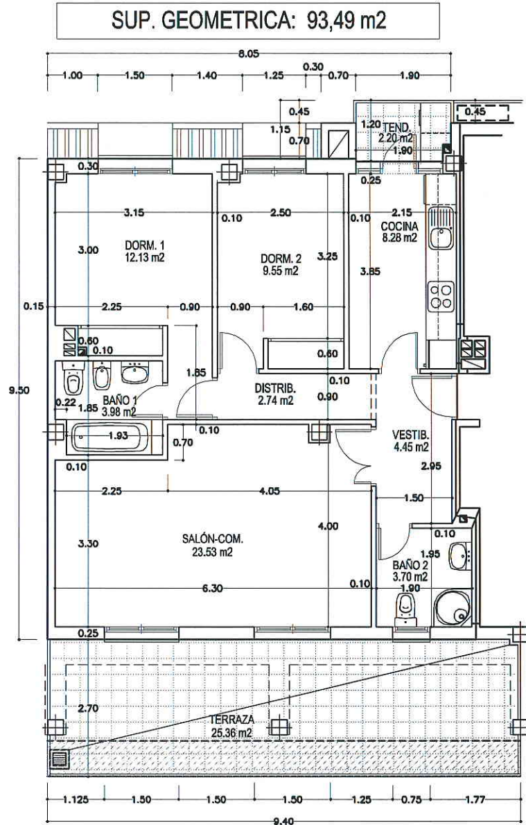
VIVIENDA TIPO 5 (5 viviendas)
